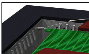
Sposób mocowania maty do konstrukcji
